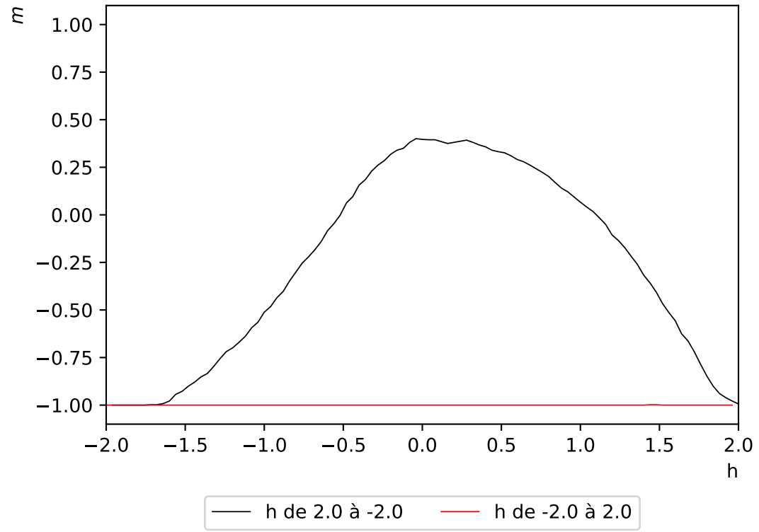
Hystérésis de l'aimantation - réseau de taille L=32 - champ magnétique d'amplitude h=2 à T=0.5
